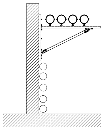
Montage de tuyauteries sur une console et une jambe de force
