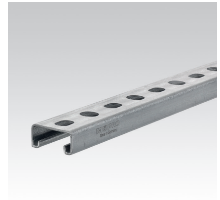
Profil 41/21/2,0
