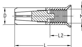
Cheville mécanique avec collerette
