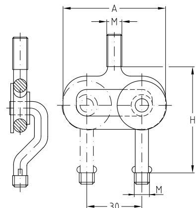
Montage d'un ensemble Fixation coulissante et collier à vis MÜPRO
